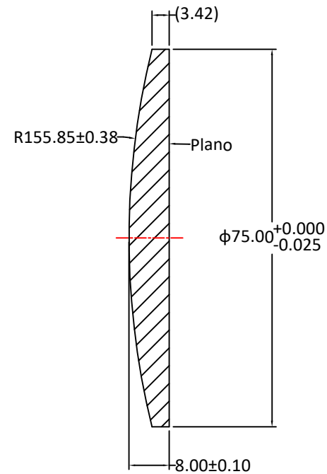
SECTION A-A
