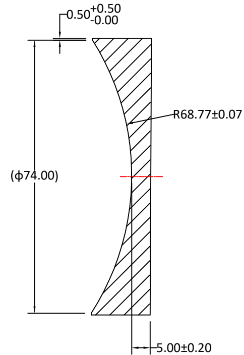
SECTION A-A
