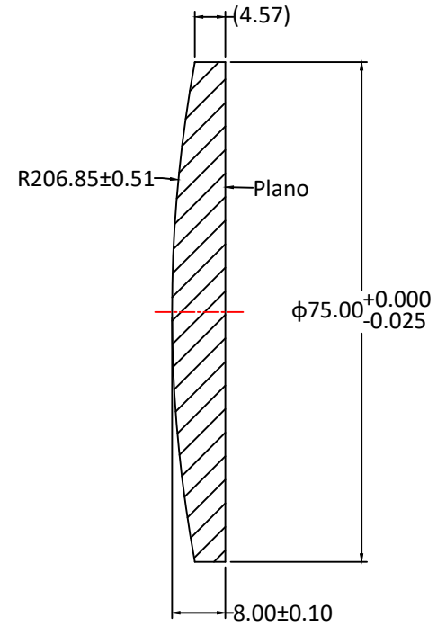
SECTION A-A
