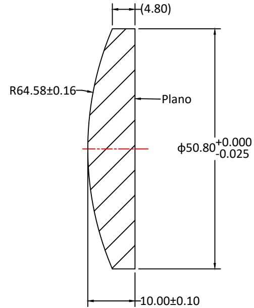
SECTION A-A
