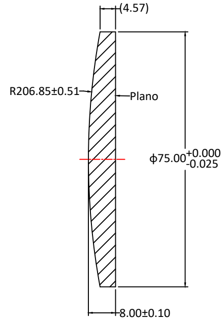
SECTION A-A
