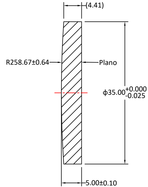
SECTION A-A
