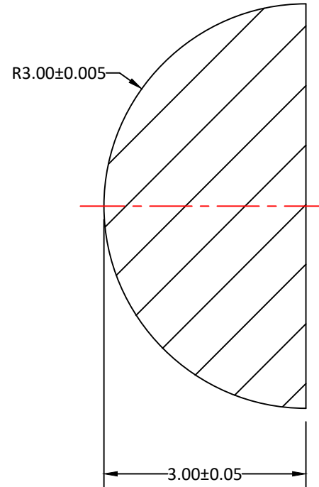
SECTION A-A
