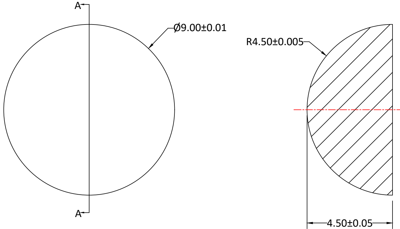
SECTION A-A
