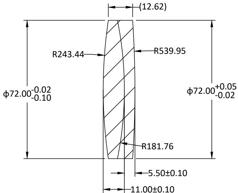
SECTION A-A
