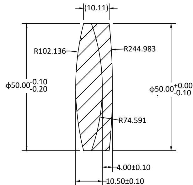
SECTION A-A
